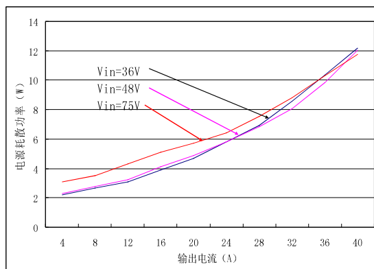
输出电流与损耗关系曲线
