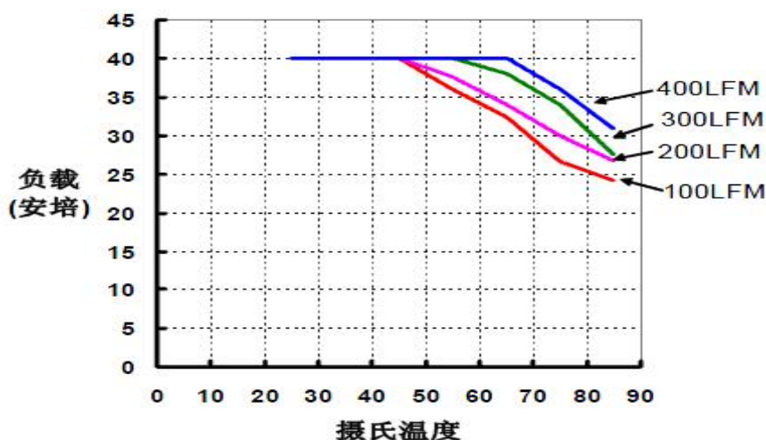
无散热器条件下的热交换曲线（不同风速条件下输出电流与环境温度的关系，Vinom）
