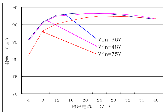
输出电流与效率关系曲线(Tc=+25℃)
